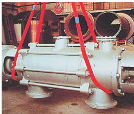
Anschlagsart: einfach umgelegt = volle Tragkraft
