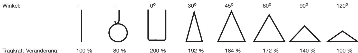
grau Tragkraft 8.000 / 4.000 kg
