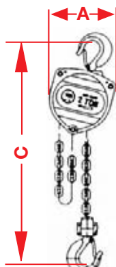
1-strängige Modelle
